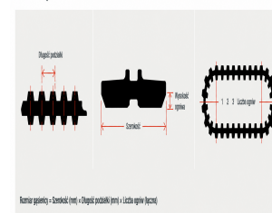
WYMIARY GĄSIENIC
