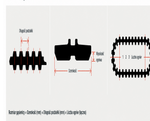
WYMIARY GĄSIENIC
