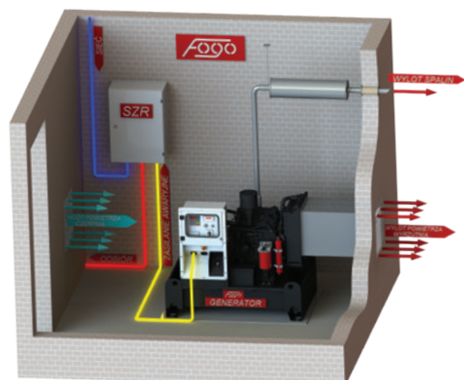
Podłączenie wewnętrzne - wersja otwarta
